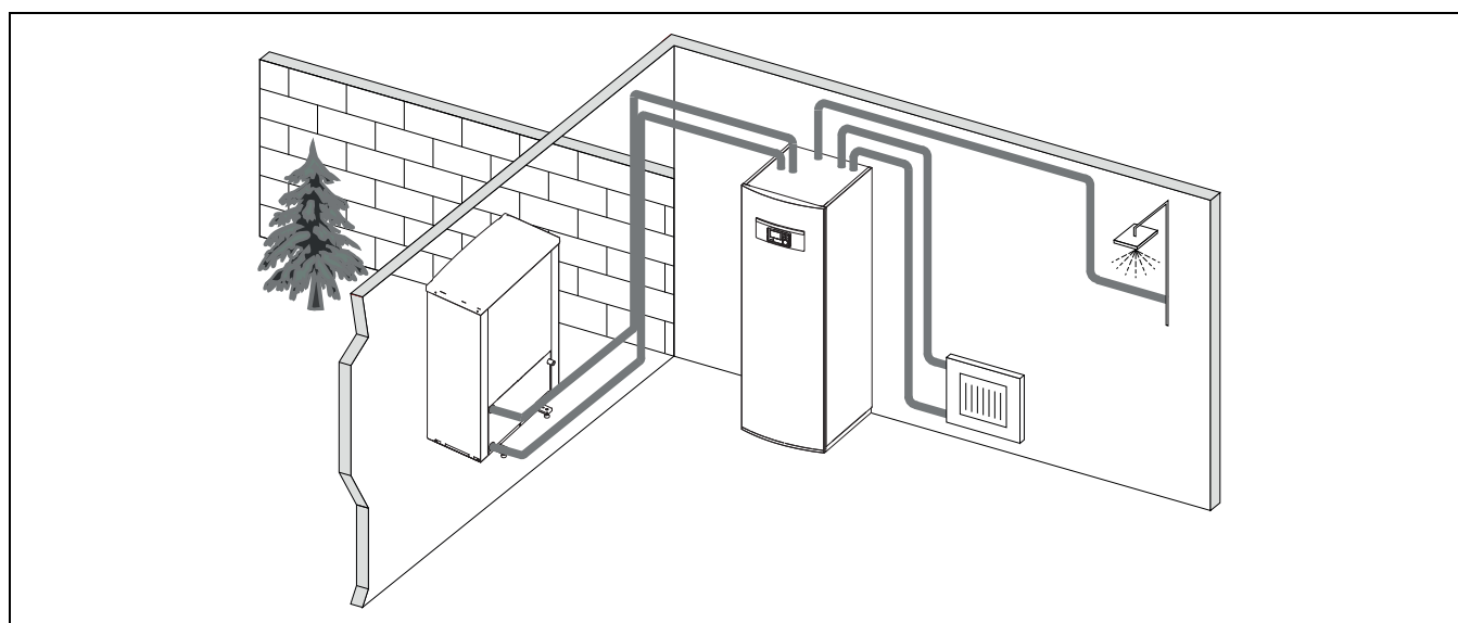
Bild 3 Värmepump AirX, inneenhet AirModule E / AirModule S/W med integrerad varmvattenberedare och eltillskott
