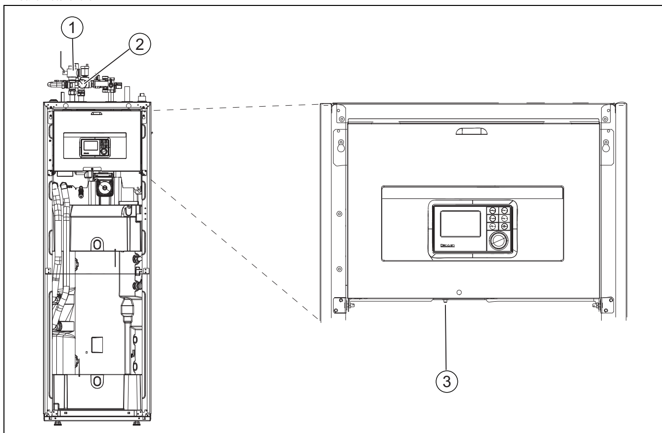
Bild 6 Inneenhet AirModule E / AirModule S/W
